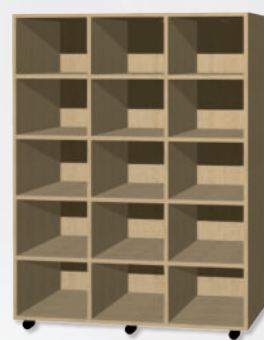
U8 REGÁL NA LOŽNÍ PRÁDLO NA KOLEČKÁCH 117 × 155 × 62 cm 15 boxů (36,5 × 27,5 × 60 cm) 9140 Kč
