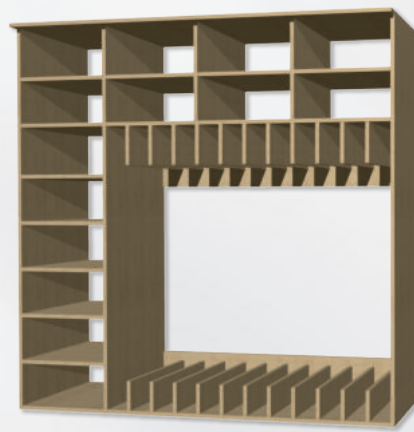
U9 STĚNA NA MATRACE A LŮŽKOVINY 200 × 200 × 62 cm + 8 cm přesah na kolejničku spodní příčky v. 15cm horní příčky v. 20cm bez zad box na lůžkoviny cca 46 × 62 × 22 cm vnitřní výška prostoru na matraci 145cm 15250 Kč (cena včetně kolejničky na závěs)
