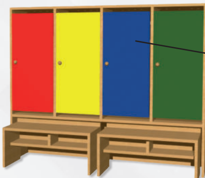
SŠ4 – ŠATNOVÁ STĚNA PRO 4 DĚTI 145 × 120 × 32 cm 7930 Kč 2 × B2 – BOTNÍK 67 × 30+3 zadní rantl × 30 cm 3160 Kč
